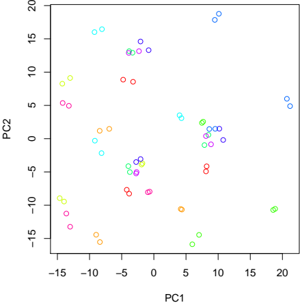
(d) hclust - colored by Individual
